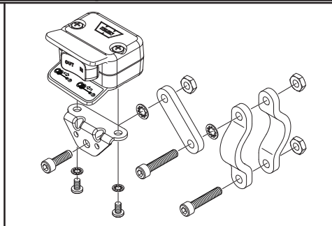
Abbildung 7: Mini-Wippenschalter.
